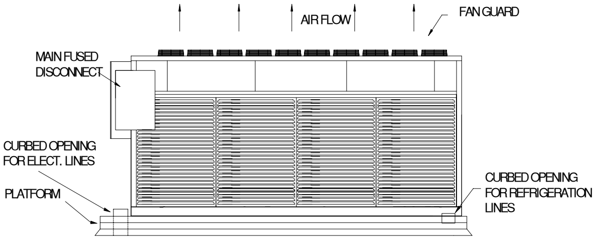
ELEVATION
